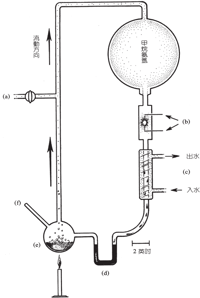
图55 米勒—尤里1953年的实验
